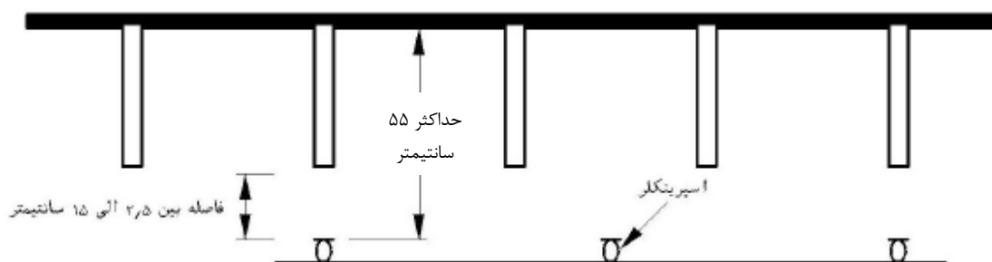
شکل ۴-۵-۱۰-الف-۱- نصب اسپرینکلر در سازه مسدودکننده
