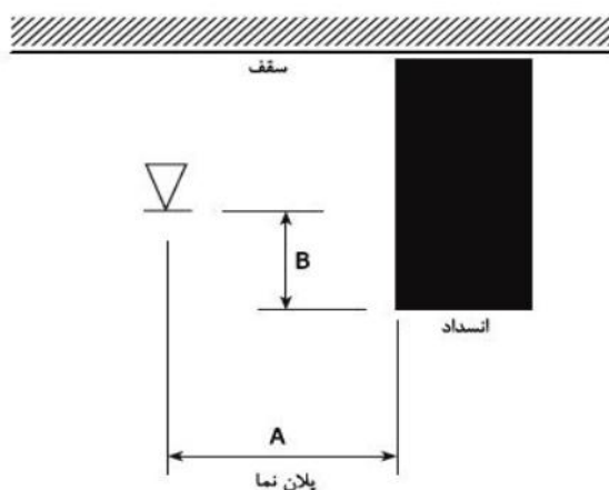
شکل ۴-۵-۱۸- فاصله اسپرینکلرها از موانع ممند نزدیک به سقف
