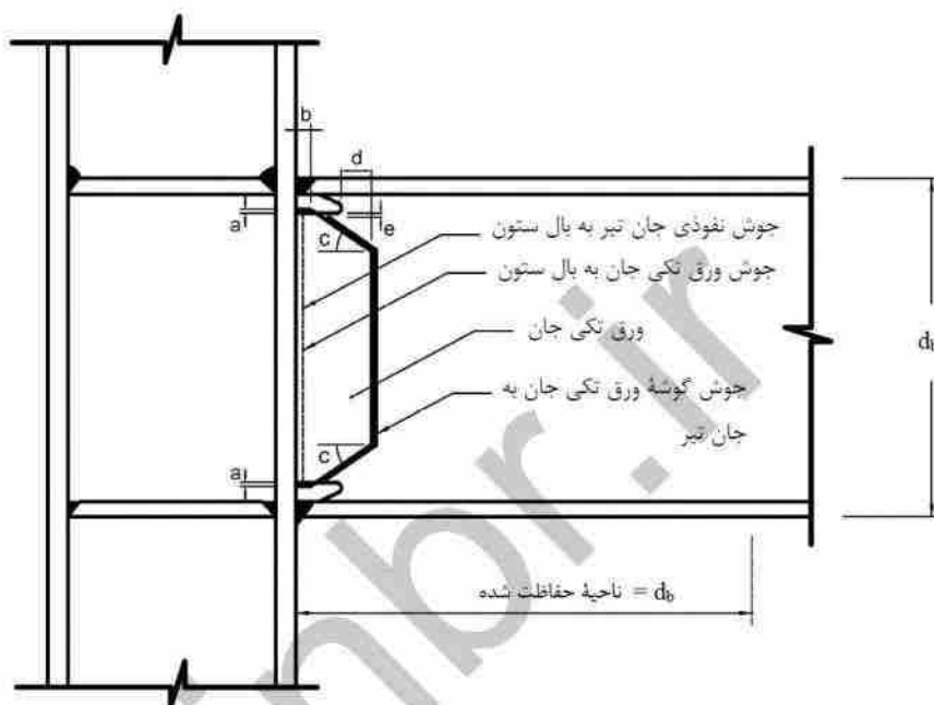
شکل ۱۰-۳-۷: اتصال گیردار تقویت نشده جوشی (WUF-W)
