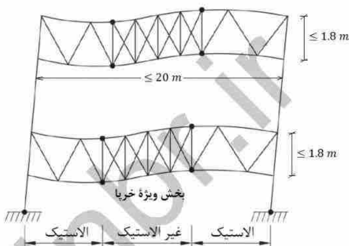
شکل ۱۰-۳-۳-۴: سازوکار تسلیم در بخش ویژه خرابا و رفتار ارتجاعی در سایر بخش‌های خرابا و ستون قاب
