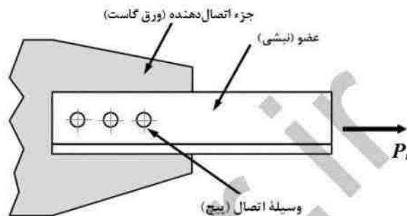
شکل ۱۰-۹-۲-۱۰: نام‌گذاری قسمت‌های مختلف یک اتصال
