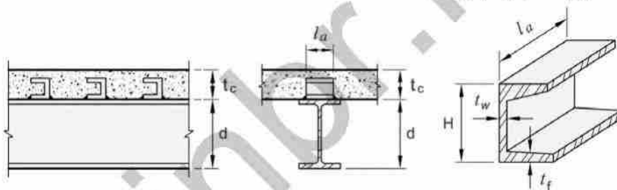
شکل ۱۰-۸-۱۷: برشگیرهای از نوع ناودانی
