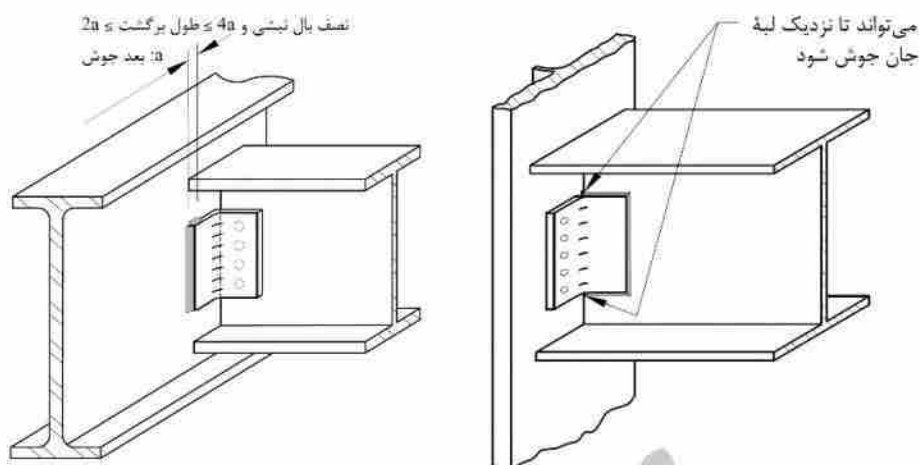
شکل ۱۰-۳-۹: اتصالات مفصلی با نبشی جان
