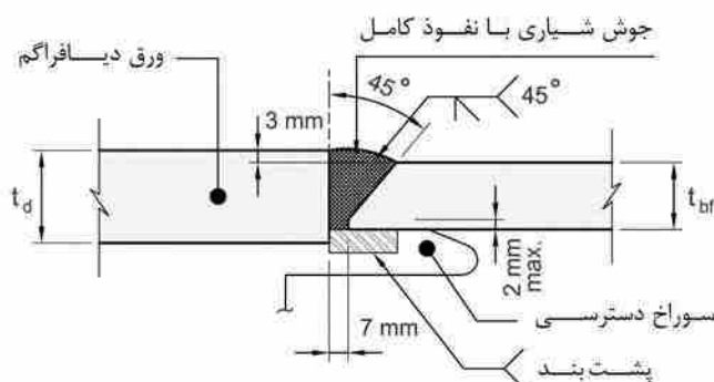
شکل ۱۰-۳-۷-۱۱: اتصال بال تیر به ورق دیافراگم با استفاده از سوراخ دسترسی و ورق‌های پشت‌بند
