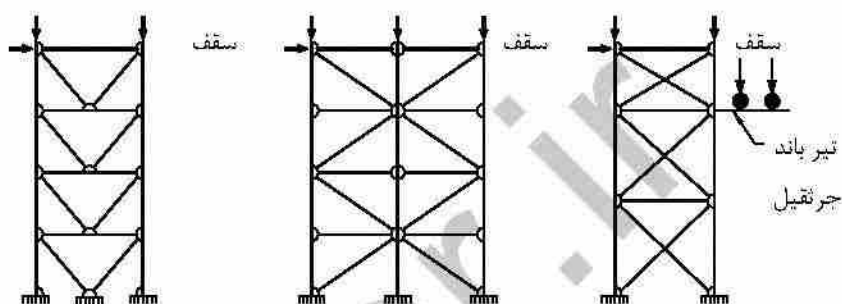
مهاربند چند ردیفی ضربدری مهاربند چند ردیفی دو دهانه مهاربند چند ردیفی از نوع ۷
