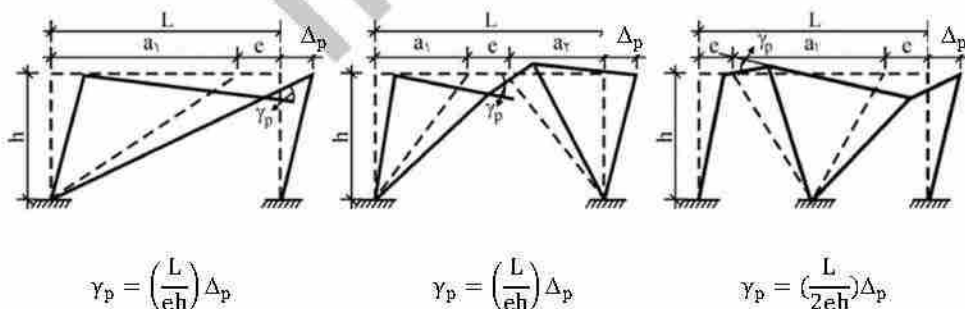
شکل ۳-۴-۳-۱۰-۲: دوران پلاستیک تیر پیوند نسبت به ناحیه خارج از آن ( \gamma_p )
