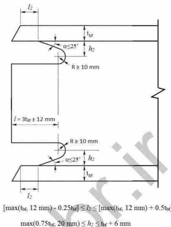
شکل ۱۰-۳-۲: دیتیل جایگزین برای سوراخ‌های دسترسی اتصالات خمشی
