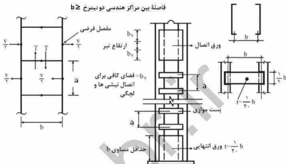
شکل ۱۰-۲-۴-۴: عضو فشاری ساخته‌شده (مرکب) با بست‌های موازی
