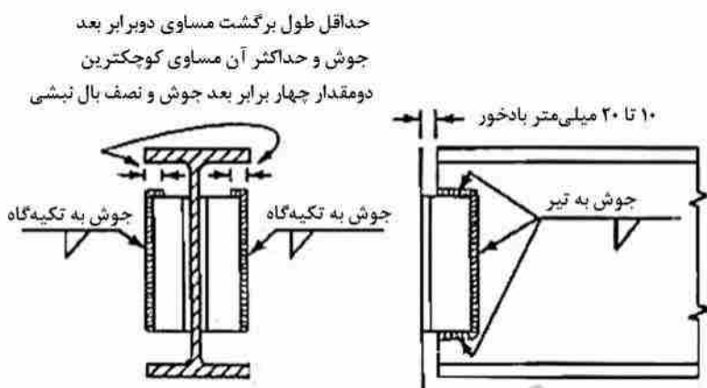
شکل ۳-۱۰-۵: جزئیات اتصال جوشی با استفاده از نبشی جفت در جان
