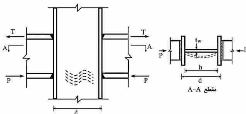
شکل ۳۹-۹-۲-۱۰: کماتش فشاری جان در مقابل یک جفت نیروی متمرکز فشاری
