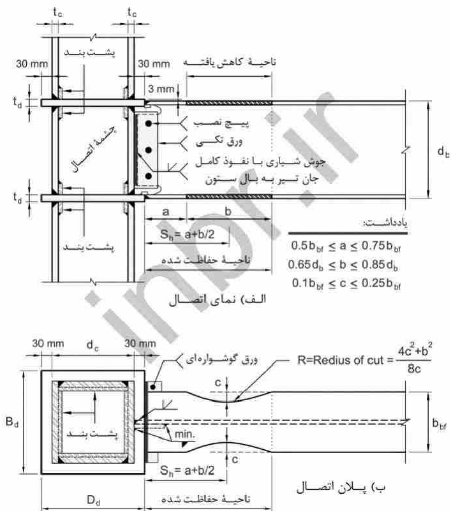
شکل ۱۰-۳-۱۰: اتصال گیردار تیر با مقطع کاهش یافته و دیافراگم عبوری از ستون (TD-RBS)
