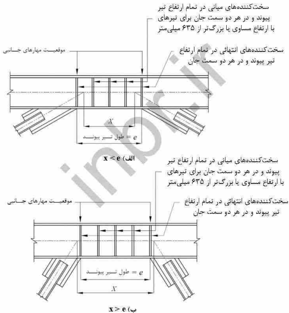
شکل ۳-۱۰-۳-۴-۲: تیر پیوند با مقطع I شکل و سخت‌کننده‌های موردنیاز
