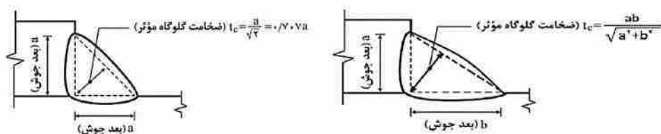
شکل ۱۰-۹-۲-۱-۱۰: بعد و ضخامت گلوگاه مؤثر جوش‌های گوشه
