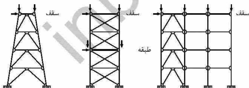
مهاربند چند ردیفی همراه با ستون‌های ثقیلی مهاربند چند ردیفی دو طبقه مهاربند چند ردیفی هرمی
