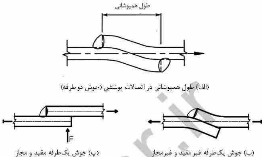
شکل ۱۰-۳-۹-۱۰: اتصال پوششی (روی هم) دو قطعه
