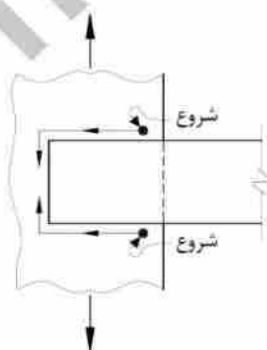
شکل ۱۰-۳-۹: مسیر مناسب برای جلوگیری از زخم (ترک یا شیار) در لبه
