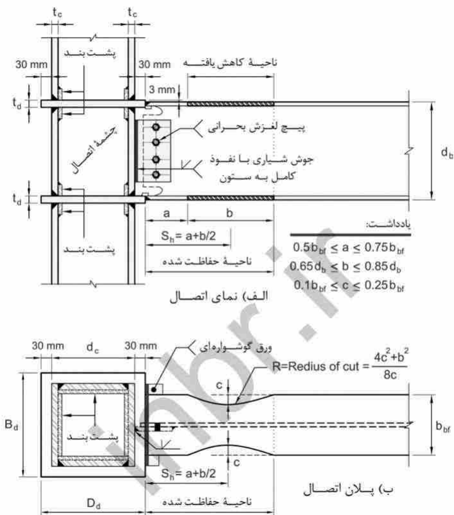
شکل ۱۰-۳-۷: اتصال گیردار تیر با مقطع کاهش یافته و دیافراگم عبوری از ستون در قاب‌های خمشی متوسط
