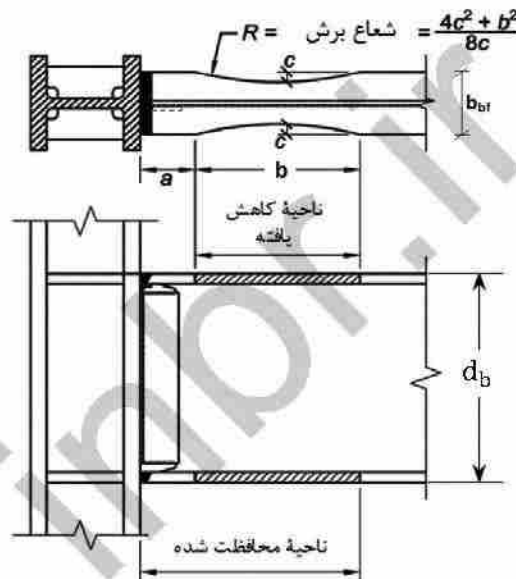
شکل ۳-۷-۳-۱۰: اتصال گیردار تیر با مقطع کاهش یافته (RBS)
