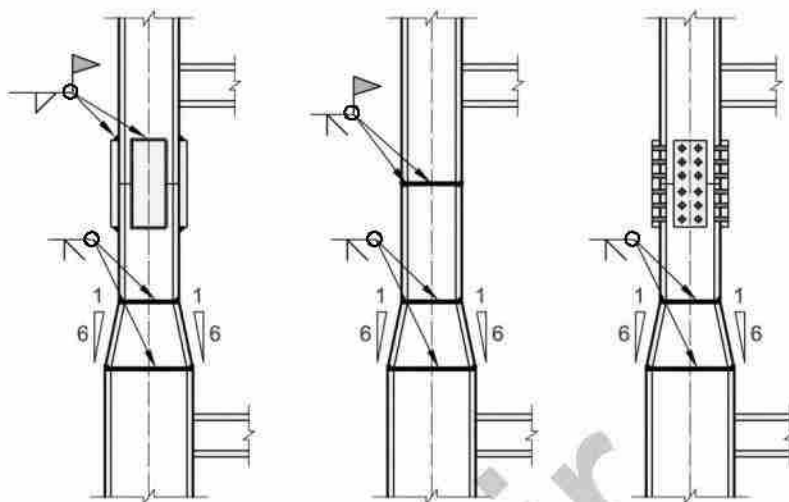
شکل ۱۰-۳-۹: جزئیات پیشنهادی وصله ستون‌ها در محل تغییر قابل ملاحظه مقطع
