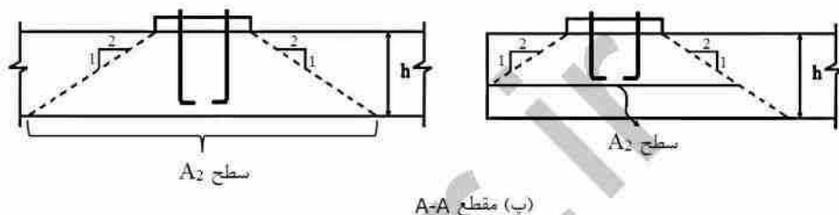
شکل ۲-۱۰-۲۲: سطح اتکا در تماس با تکیه‌گاه بتنی
