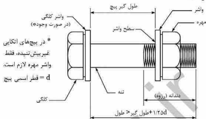
شکل ۴-۱۰-۳: اجزای مختلف پیچ و مهره
