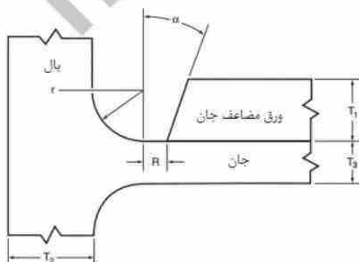
شکل ۱۰-۴-۲۷: جزئیات اتصال ورق مضاعف جان به مقاطع نورددشه
