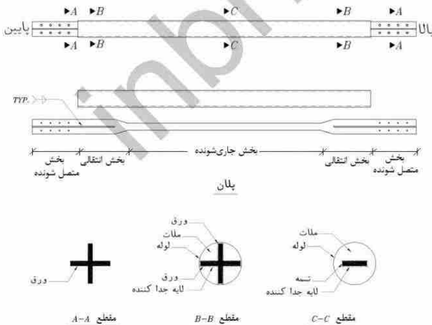
شکل ۱۰-۳-۴-۴-۱: نمونه‌ای از اجزای یک مهاربند کمانش تاب
