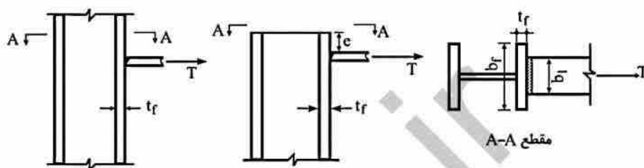
شکل ۲-۱۰-۹-۳-۱۰: خمش موضعی بال در مقابل نیروی متمرکز کششی
