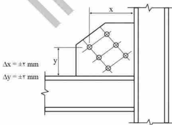
شکل ۴-۱۰-۲۱: رواداری مختصات سوراخ پیچ‌ها نسبت به مختصات مقرر در نقشه‌ها
