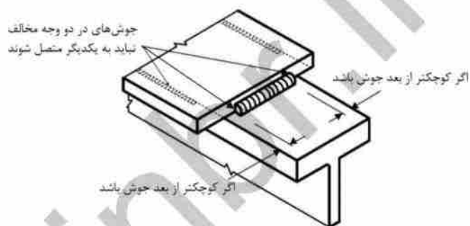
شکل ۱۰-۳-۹: جوش های گوشه در دو وجه مخالف یک صفحه مشترک
